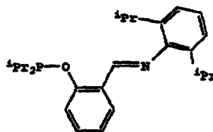
N-(ortho-diisopropylphosphinoxy)benzyl-2,6-diisopropylanilineimine
