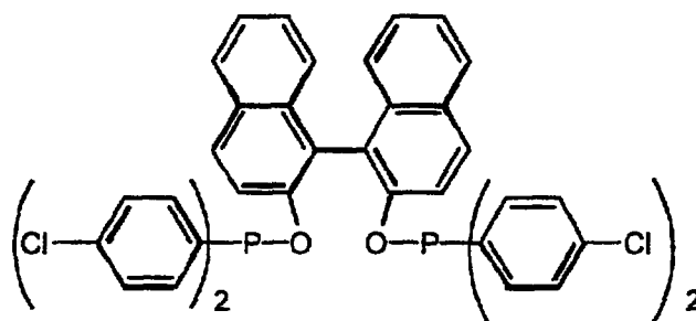
Ligand G
