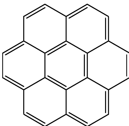
coronene
