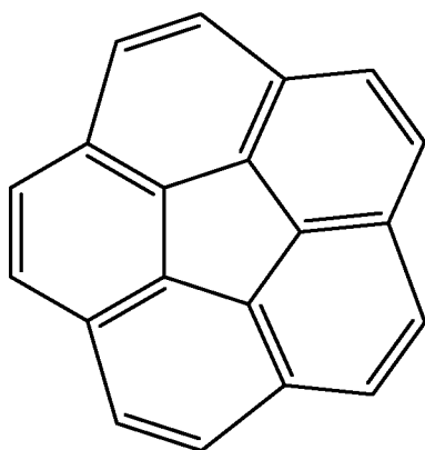
corannulene
