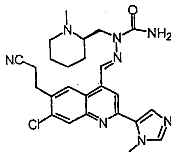
R-(+) (R)-(+) -6
