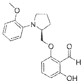
(S)-2-hydroxy-6-((1-(2-methoxyphenyl)pyrrolidin-2-yl)methoxy)benzaldehyde
