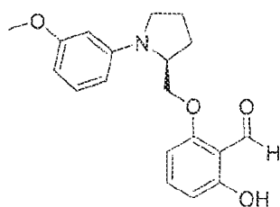
(S)-2-hydroxy-6-((1-(3-methoxyphenyl)pyrrolidin-2-yl)methoxy)benzaldehyde
