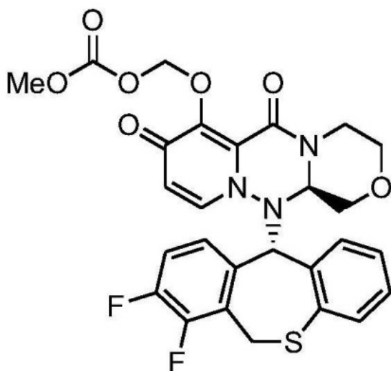
(Baloxavir Marboxil)
