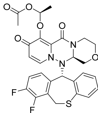
(I-1-1-1)
