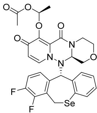
(I-1-1-4)
