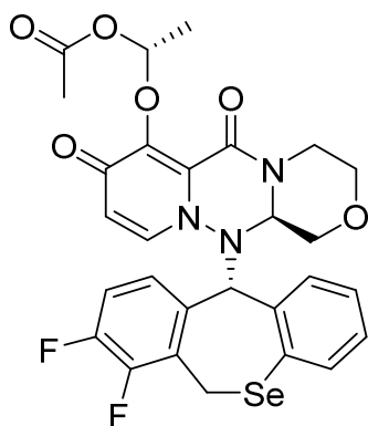
(I-1-1-5)
