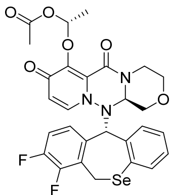
(I-1-1-5)
