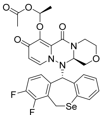
(I-1-1-4)
