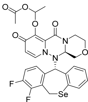
(I-1-1-6)
