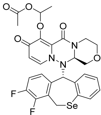
(I-1-1-6)
