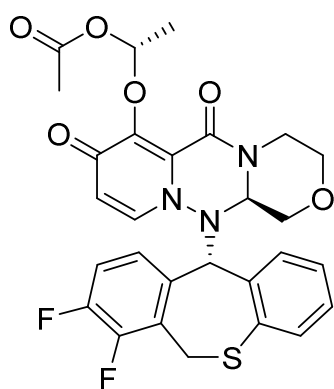
(I-1-1-1)
