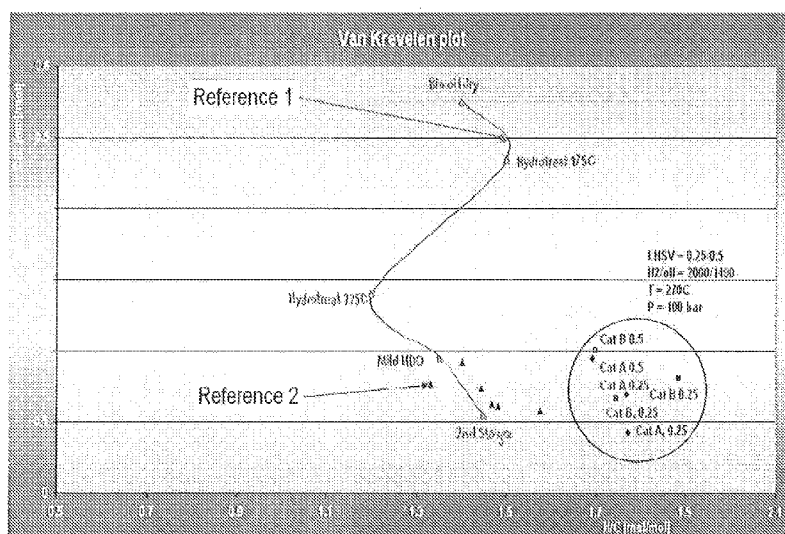
Van Krevelen plot: Cat A/Cat B
