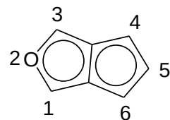
cyclopenta[c]furyl
