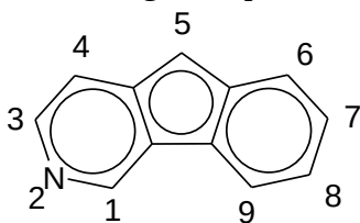
indeno[1,2-c]pyridyl
