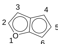
cyclopenta[b]furyl
