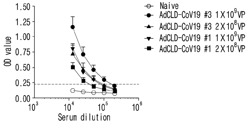
AdCLD-CoV19 마우스 혈청 2~4주차 ELISA
