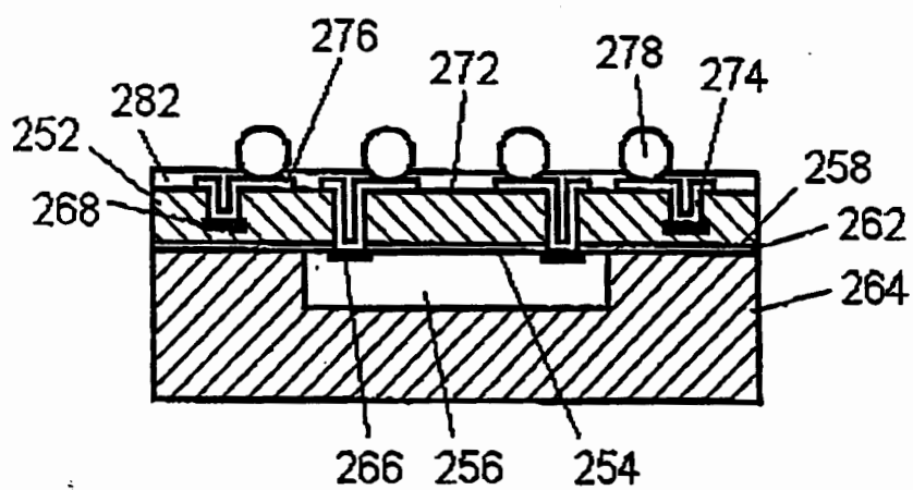
FIG. 29. PRIOR ART
