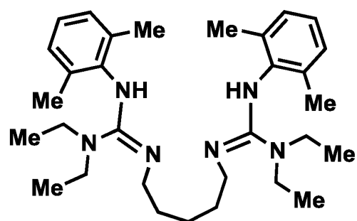
Ligand 16
