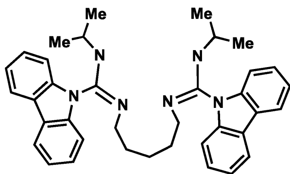
Ligand 15
