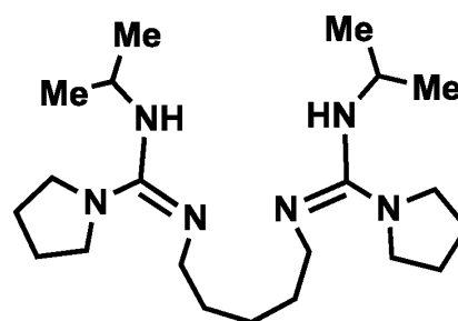
Ligand 12
