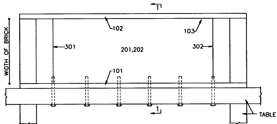
ELEVATION
