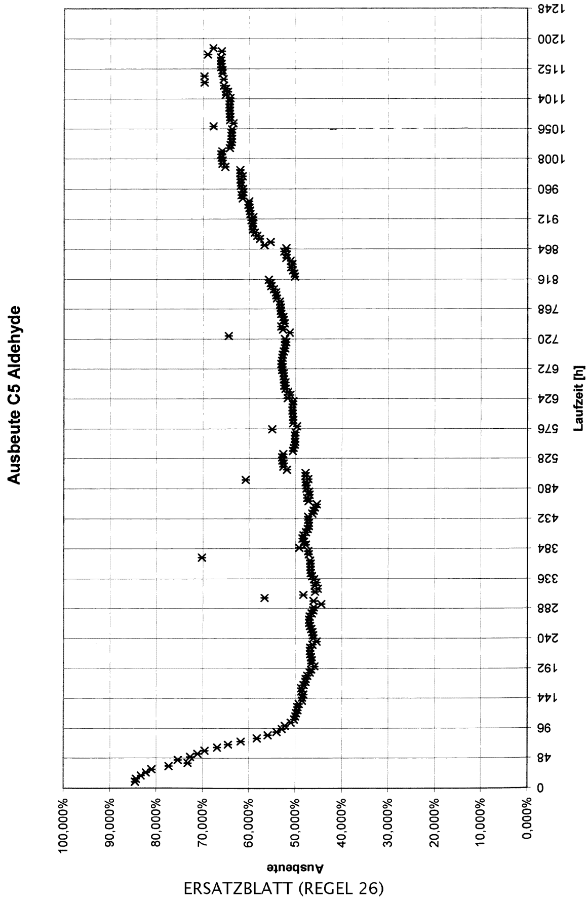
Fig. 2 (Stand der Technik)
