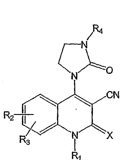
(IVa)
