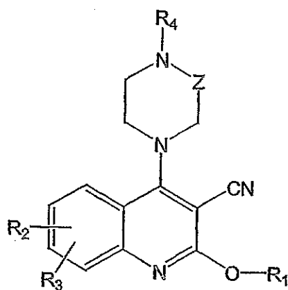
(VIIb)
