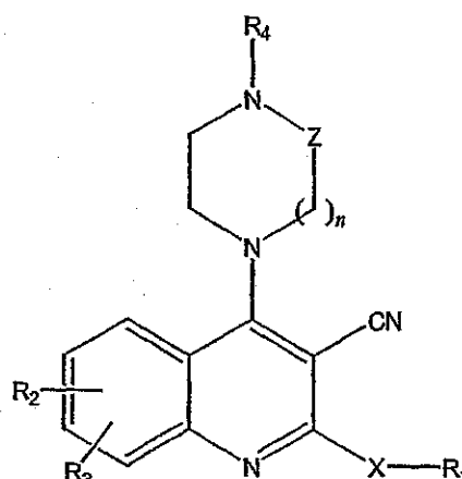
(Ib)
