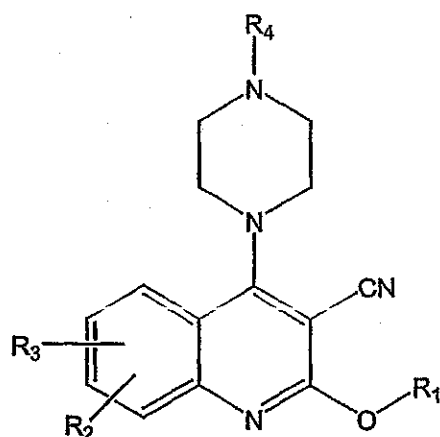
(Formula IVb)
