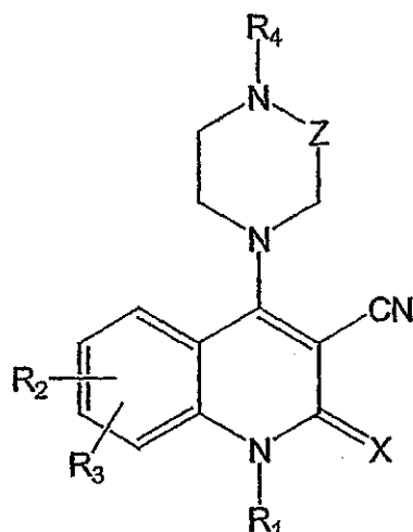
(Va)
