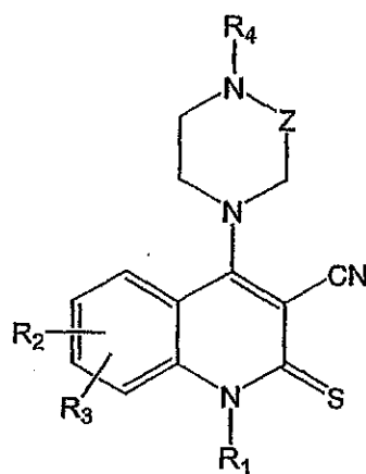
(VIIIa)
