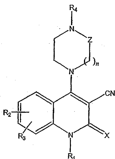
(Ia)
