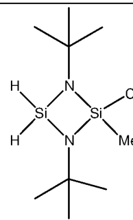
1,3-bis(tert-butyl)-2-chloro-2-methylcyclodisilazane
