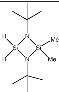
1,3-bis(tert-butyl)-2-dimethylcyclodisilazane
