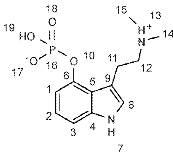
Psilocybin
