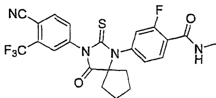
RD162" (Formula 44)
