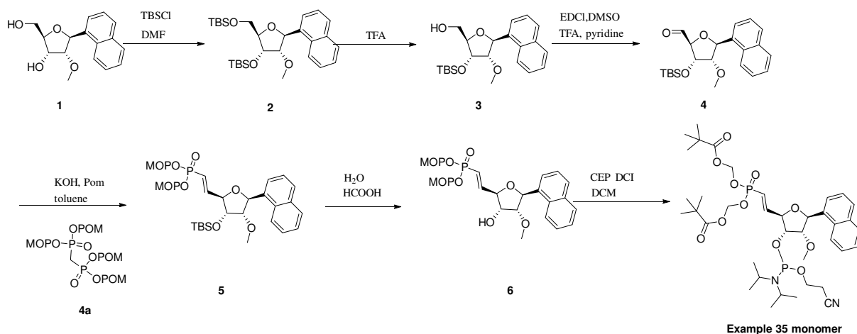
Scheme-15
