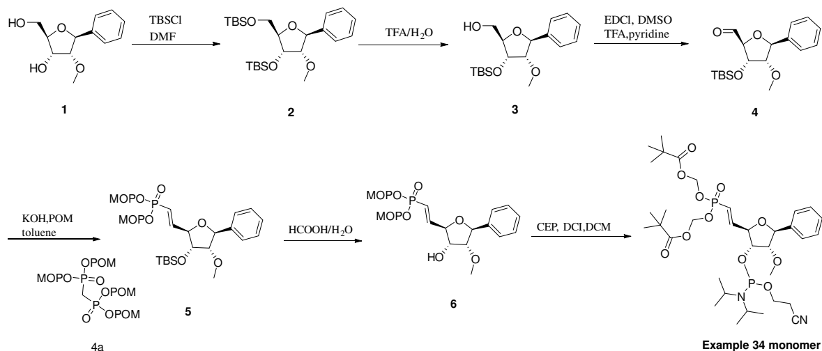
Scheme-14
