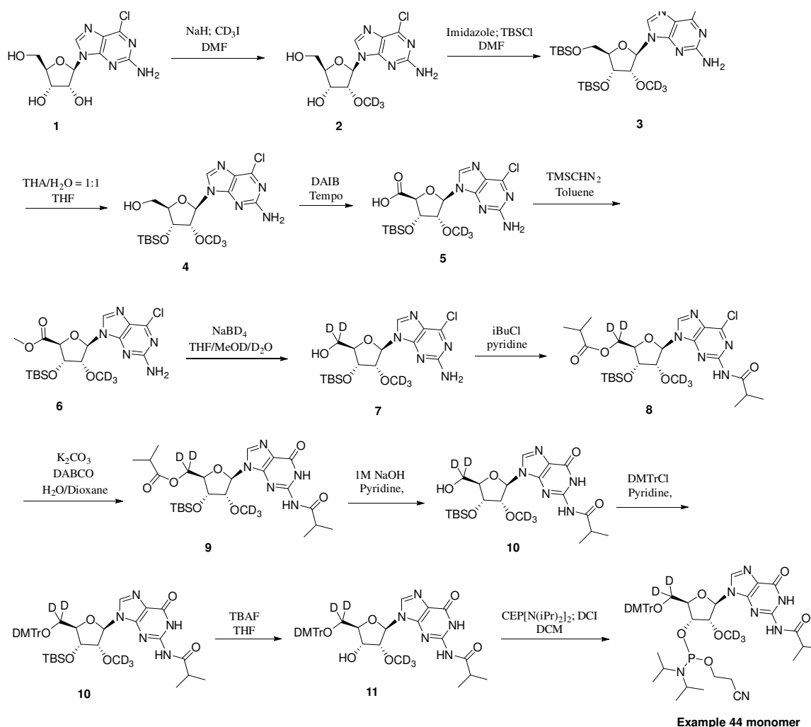
Scheme-24
