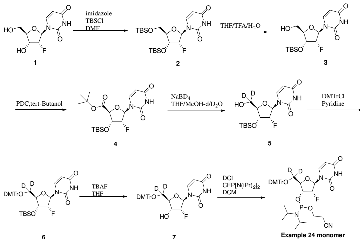
Scheme-4
