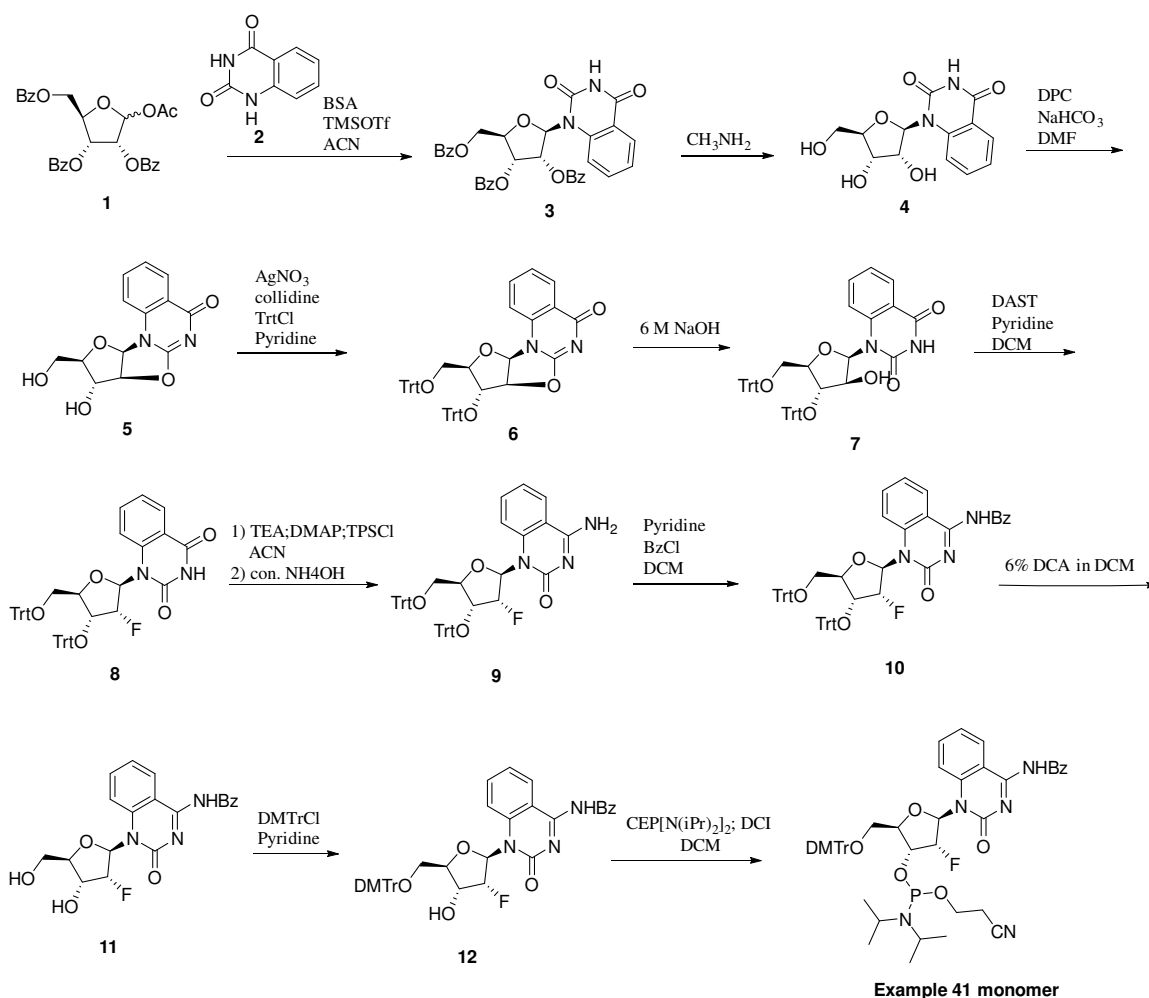
Scheme-21
