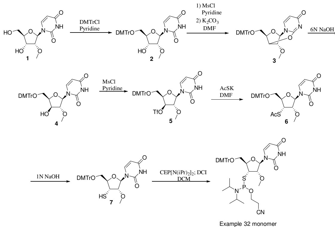
Scheme-12
