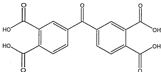
(benzophenone-3,3',4,4'—tetracarboxylic acid)
