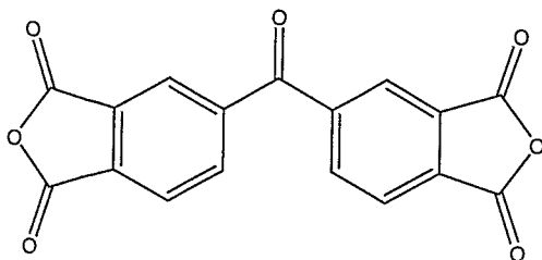
(benzophenone-3,3',4,4'—tetracarboxylic dianhydride)
