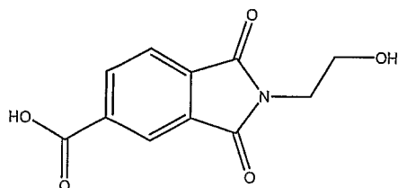
(HETI)
