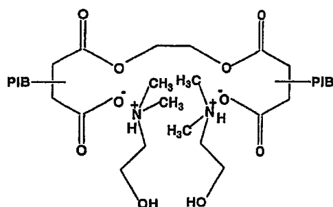
PIBSA:EG:DMEA ( \approx 2:1:2 (eq))
