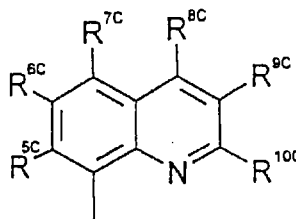
8-quinolyl
