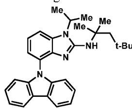
Ligand 33
