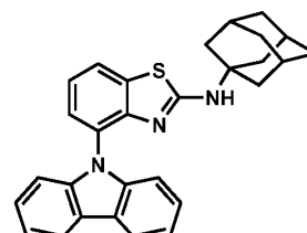
Ligand 18
