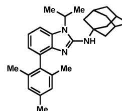
Ligand 30
