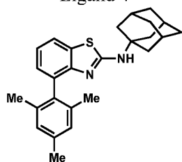
Ligand 7
