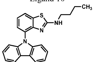
Ligand 13
