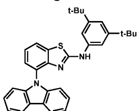
Ligand 20
