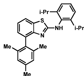
Ligand 12
