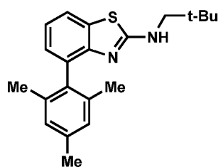
Ligand 2
