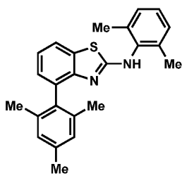
Ligand 11
