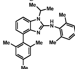
Ligand 32
