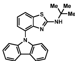
Ligand 17
