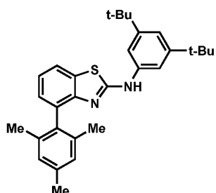
Ligand 10
