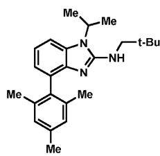
Ligand 26
