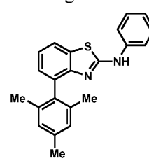
Ligand 9
