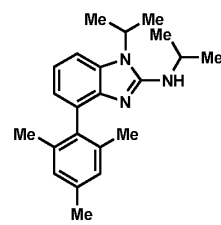
Ligand 27
