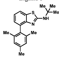
Ligand 6
