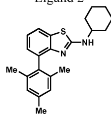
Ligand 5
