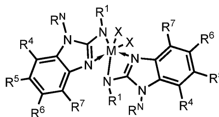
(IIId)
