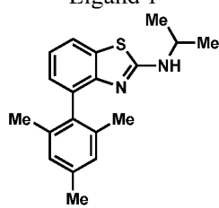
Ligand 4
