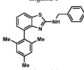
Ligand 8
