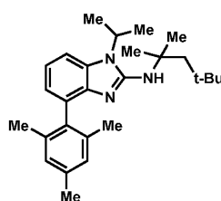
Ligand 29
