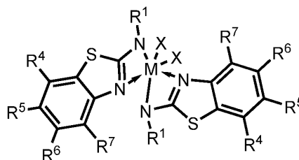
(IIb)
