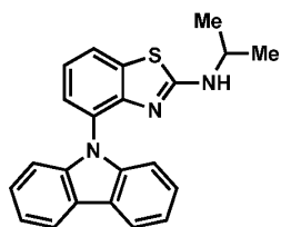
Ligand 16
