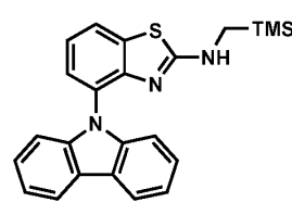
Ligand 15
