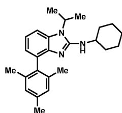
Ligand 28
