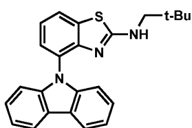
Ligand 14
