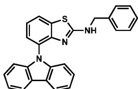
Ligand 19
