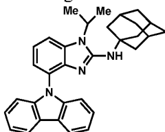
Ligand 34
