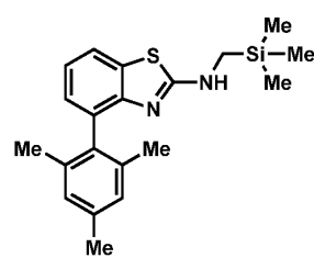
Ligand 3
