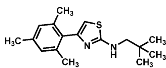
Ligand 23
