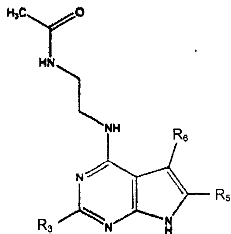
VII
