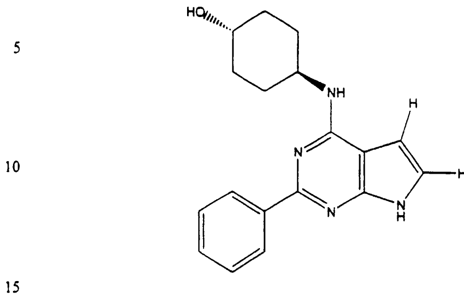
(Compound 1318-a)
