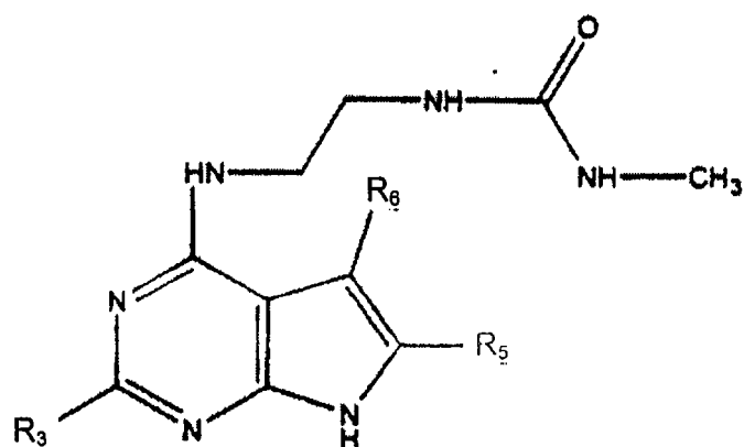
VIII
