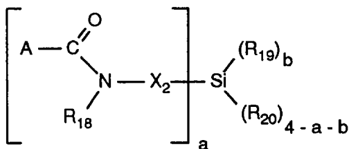
(VIa)
