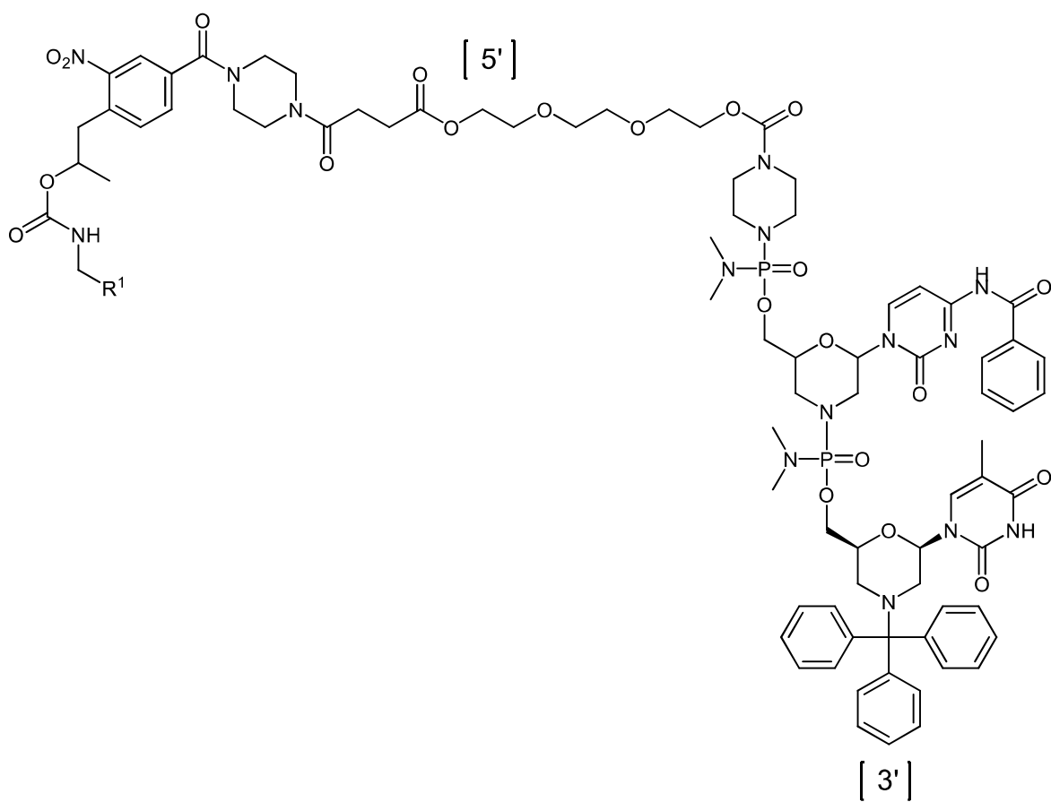
(VIIa),
