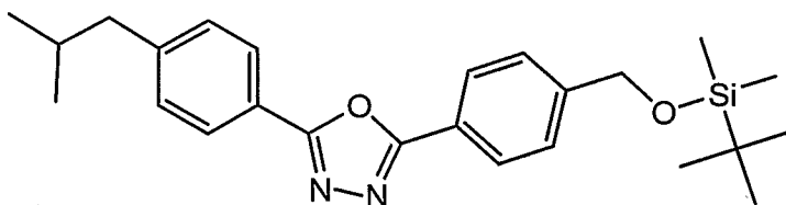
9D: 2-[4-({[tert-Butyl(dimethyl)silyl]oxy}methyl)phenyl]-5-(4-isobutylphenyl)-1,3,4-oxadiazole
