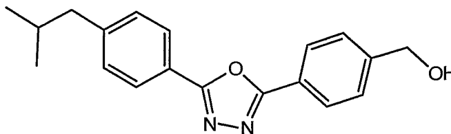
9E: {4-[5-(4-Isobutylphenyl)-1,3,4-oxadiazol-2-yl]phenyl}methanol
