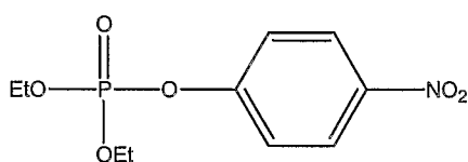
Paraoxon
