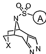
Formula VIIb
