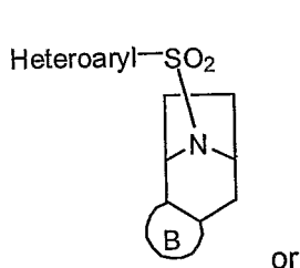
Formula Va
