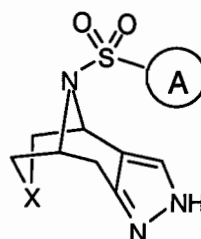
Formula VIIb
