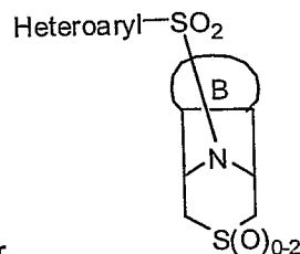
Formula Vf
