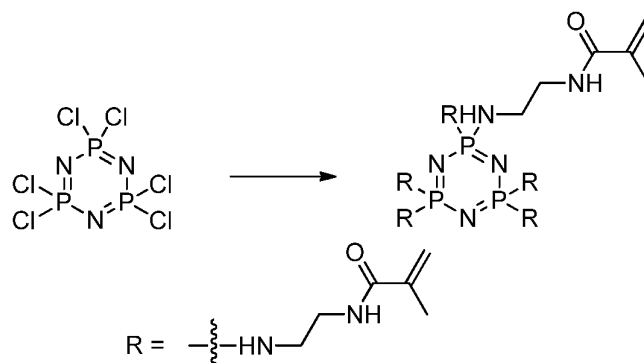
Scheme 10.1.
