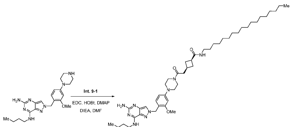
(1s,3s)-3-(2-(4-(4-((5-amino-7-(butylamino)-2H-pyrazolo[4,3-d]pyrimidin-2-yl)methyl)-3-methoxyphenyl)piperazin-1-yl)-2-oxoethyl)-N-octadecylcyclobutane-1-carboxamide (B-9)
