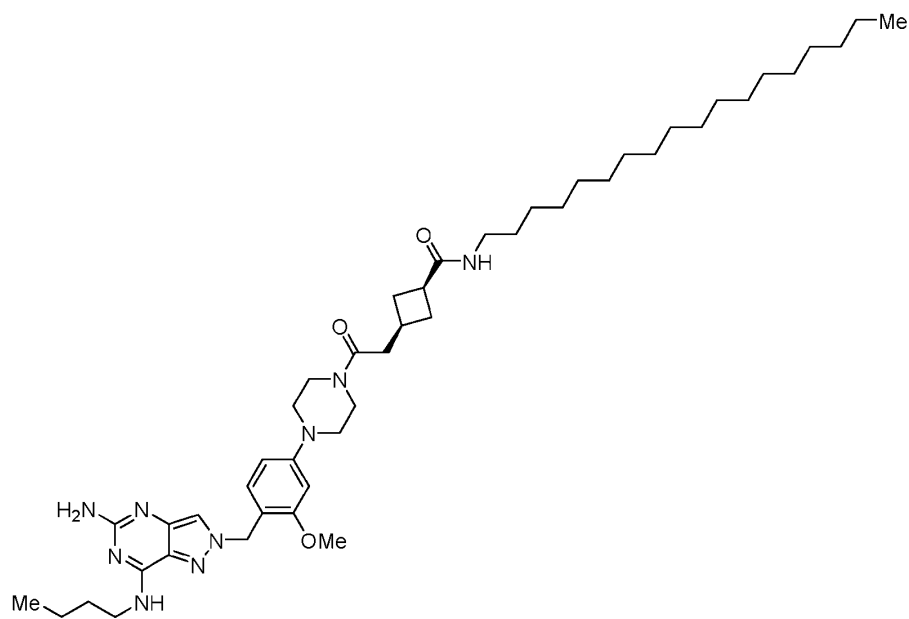
(1s,3s)-3-(2-(4-(4-((5-amino-7-(butylamino)-2H-pyrazolo[4,3-d]pyrimidin-2-yl)methyl)-3-methoxyphenyl)piperazin-1-yl)-2-oxoethyl)-N-octadecylcyclobutane-1-carboxamide (B-9)
