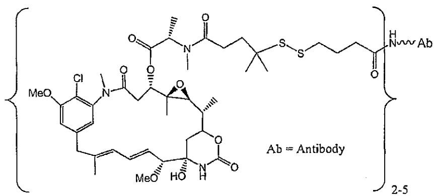
Ab-SPDB-DM4
