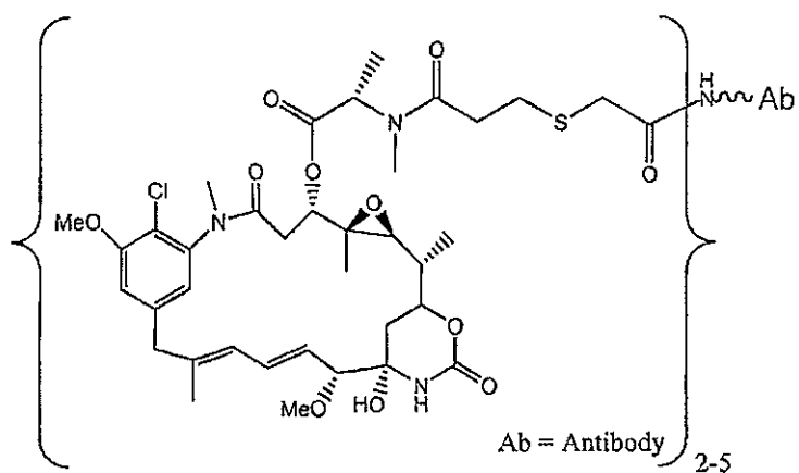
Ab-SIA-DM1
