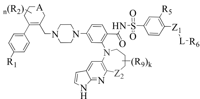
Formula (D)
