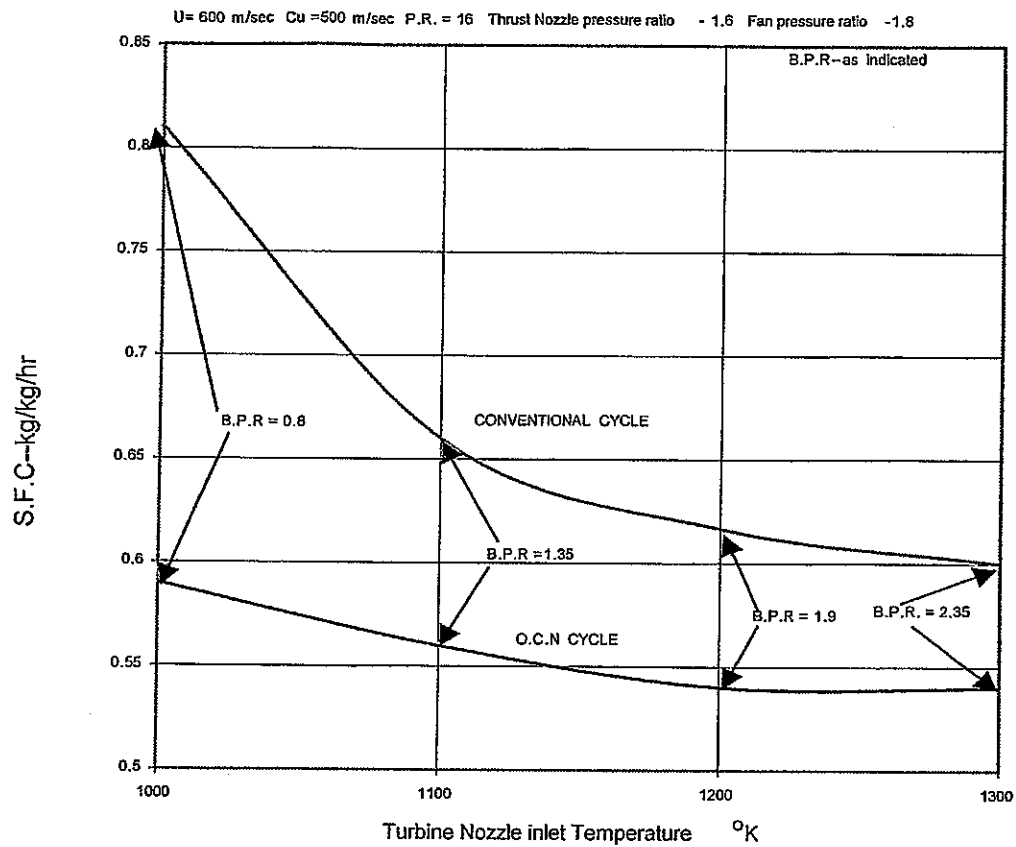
Fig 7. O.C.N TURBOFAN S.F.C.
