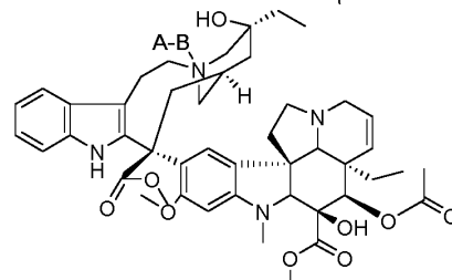
Vinblastine
