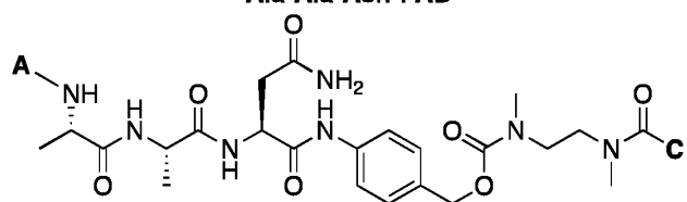
Ala-Ala-Asn-PAB
