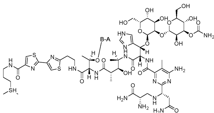
Bleomycin A2
