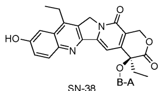
SN-38
