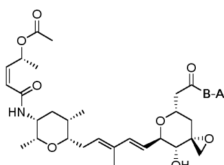
thailanstatin A
