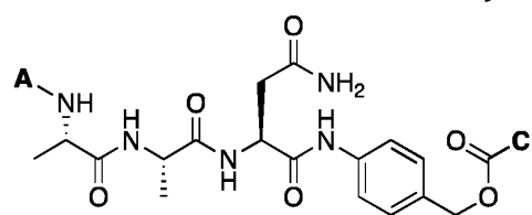
Ala-Ala-Asn-PAB
