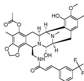
PM00104
