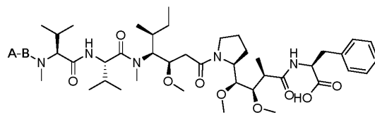
AS269
