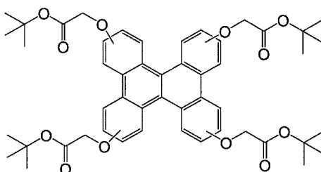
(HDBC-4-MeBOC)
