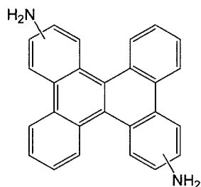
(NH 2 DBC-2)
