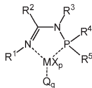
Structure NPAMC1
