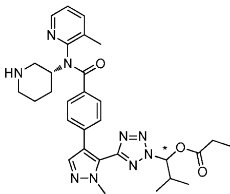
(Diastereomer A)
