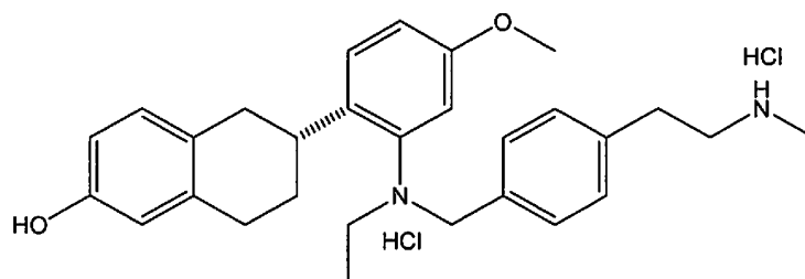
RAD1901-2HCl
