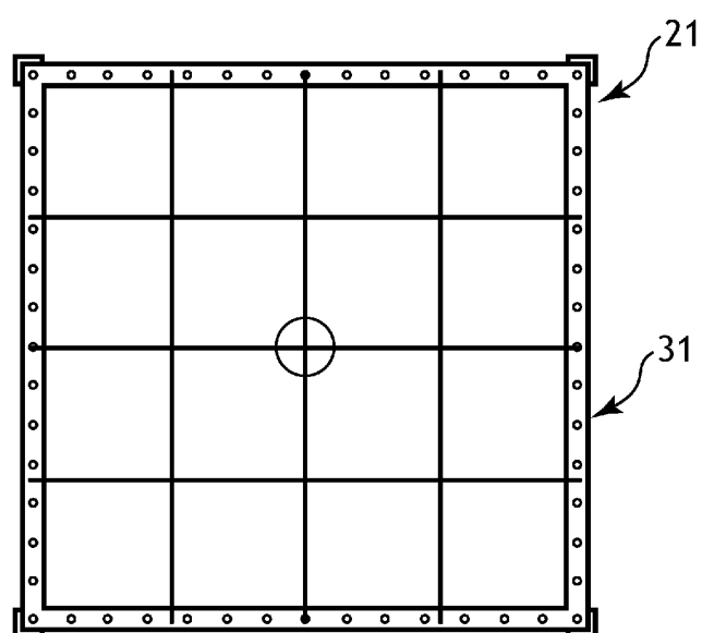
[平面図]
