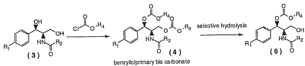
FIG. 3A (Scheme 5)
