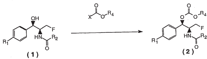
FIG. 3B (Scheme 6)
