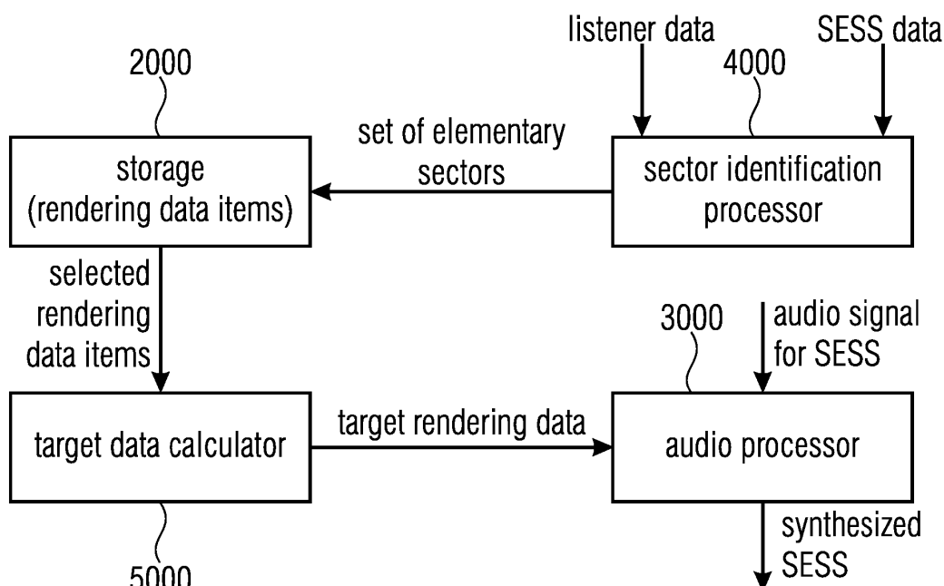
Fig. 1 (FIRST ASPECT)
