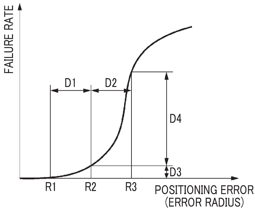
8/8 FIG. 9
