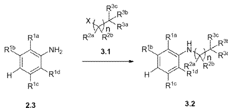
Scheme 3A.
