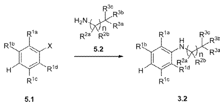
Scheme 5A.
