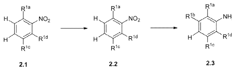
Scheme 2A.
