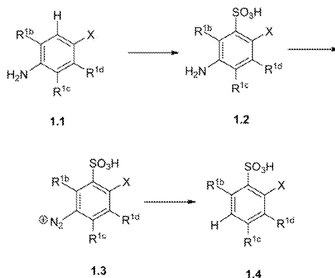
Scheme 1A.
