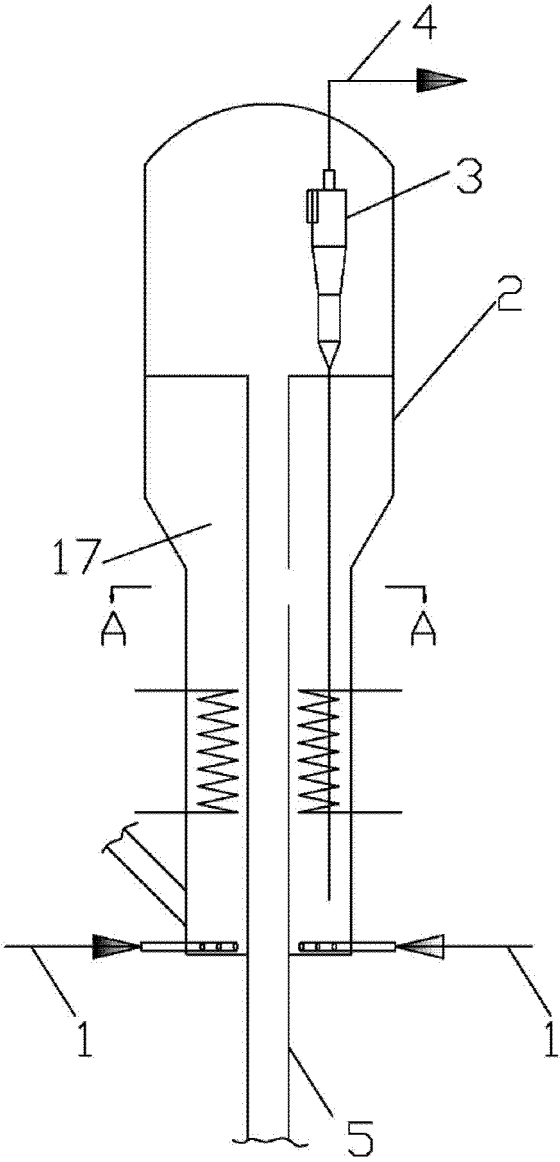
A-A剖面
