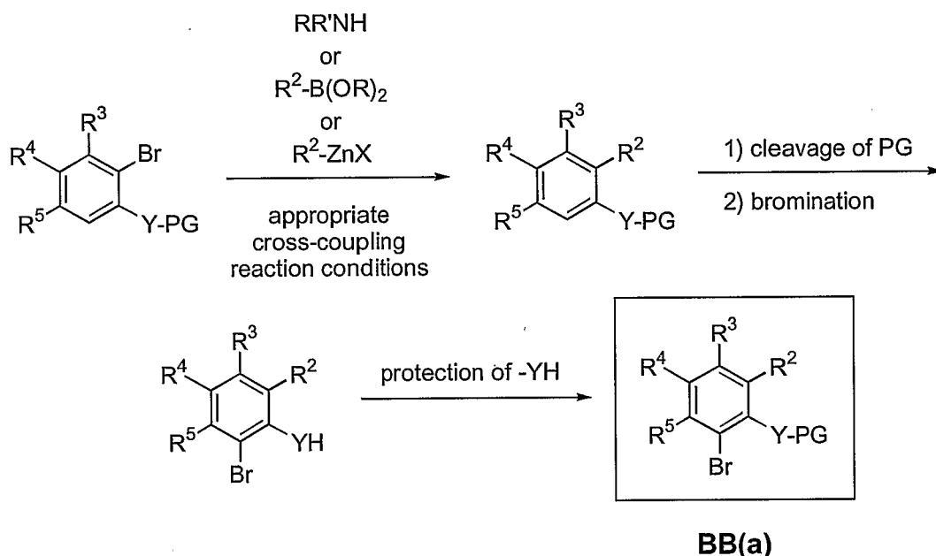
Scheme 1a
