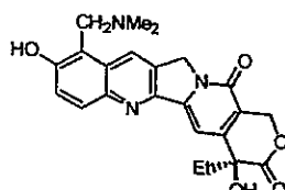
topotecan (tpi)
