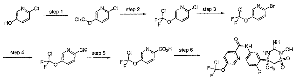
Ex. 122
