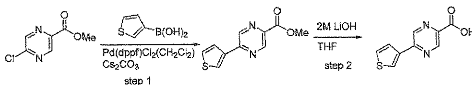
Scheme 11e:
