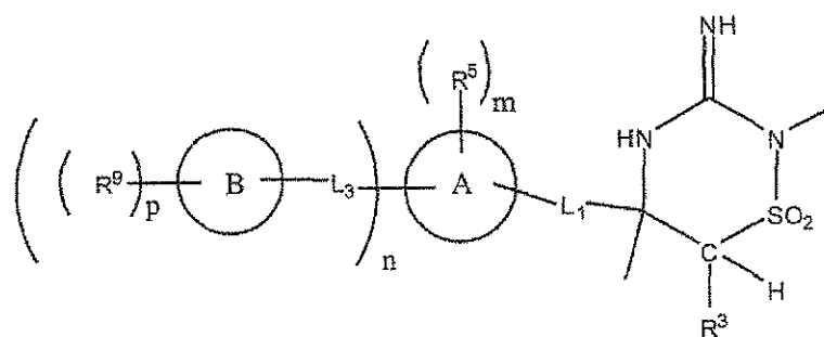
(II).
