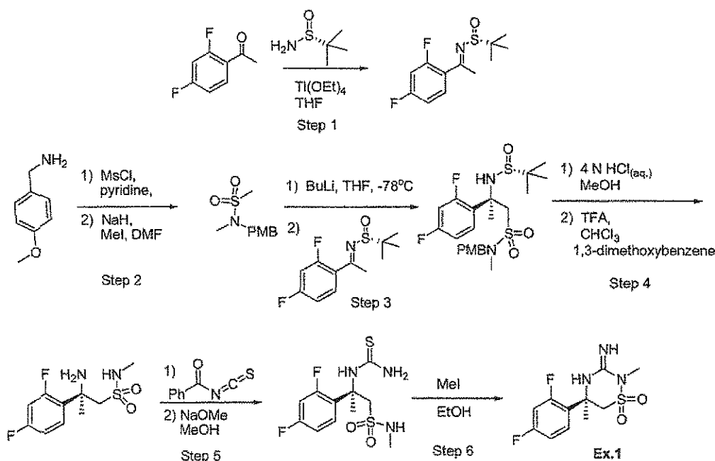
Scheme 1a
