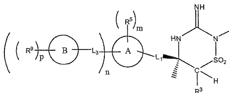
(IIA)
