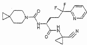
N-[(S)-1-(1-cyanocyclopropylcarbamoyl)-4,4-difluoro-4-pyridin-3-ylbutyl]-6-azaspiro[2.5]octane-6-carbonsäure
