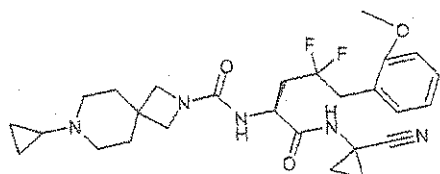
N-[(S)-1-(1-cyanocyclopropylcarbamoyl)-3,3-difluoro-4-(2-fluorophenyl)butyl]- 7-cyclopropyl-2,7-diazaspiro[3.5]nonane-2-carboxamide
