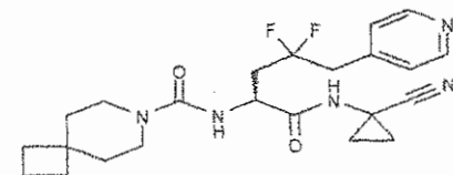
15 N-[(S)-1-(1-cyanocyclopropylcarbamoyl)-3,3-difluoro-4-(2-methoxyphenyl)butyl]-7-cyclopropyl-2,7-diazaspiro[3.5]nonane-2-carboxamide
