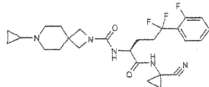
N-[(S)-1-(1-cyanocyclopropylcarbamoyl)-4-(2-difluoromethoxyphenyl)-4,4-difluorobutyl]-7-cyclopropyl-2,7-diazaspiro[3.5]nonane-2-carboxamide
