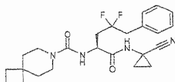
5 N-[(S)-1-(1-cyanocyclopropylcarbamoyl)-3,3-difluoro-4-pyridin-2-ylbutyl]-7-azaspiro[3.5]nonane-7-carboxamide
