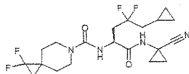
N-[(S)-1-(1-cyanocyclopropylcarbamoyl)-3,3-difluoro-4-pyridin-3-ylbutyl]-1,1-difluoro-6-azaspiro[2.5]octane-6-carboxamide
