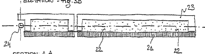
SECTION A-A Fig. 3C
