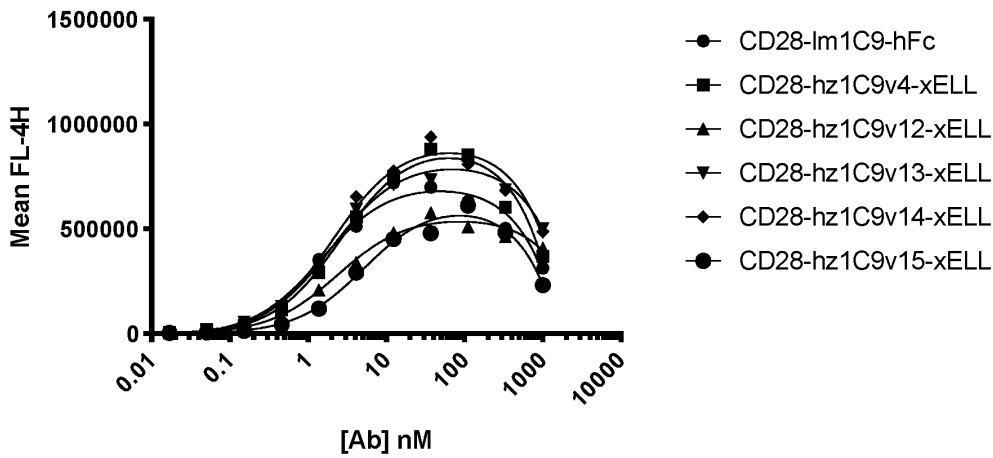
Fig. 2E cyCD28-293FS
